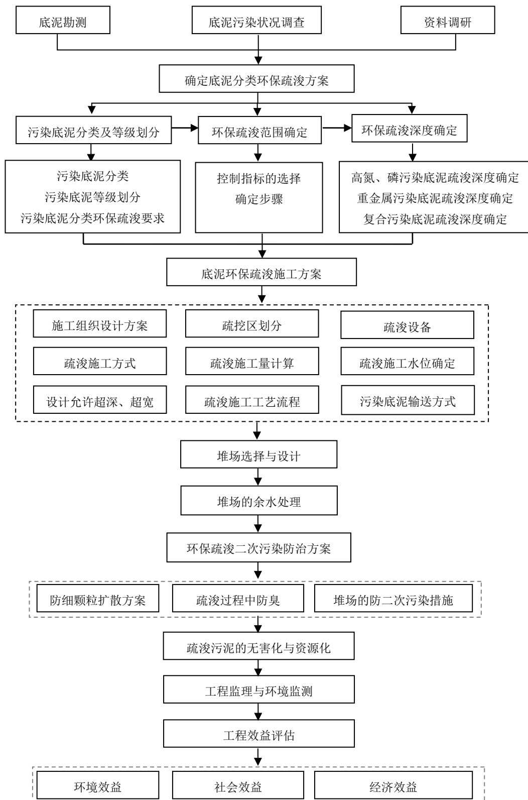
图 2-1 污染底泥环保疏浚工程方案设计技术路线
