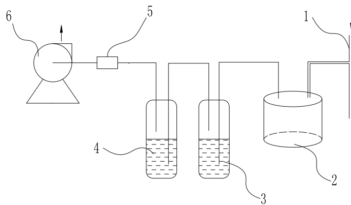
图 3-4 田间原位测定氨挥发的装置
