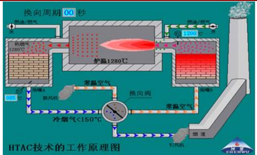
图5：神雾集团蓄热式高温空气燃烧技术原理图
