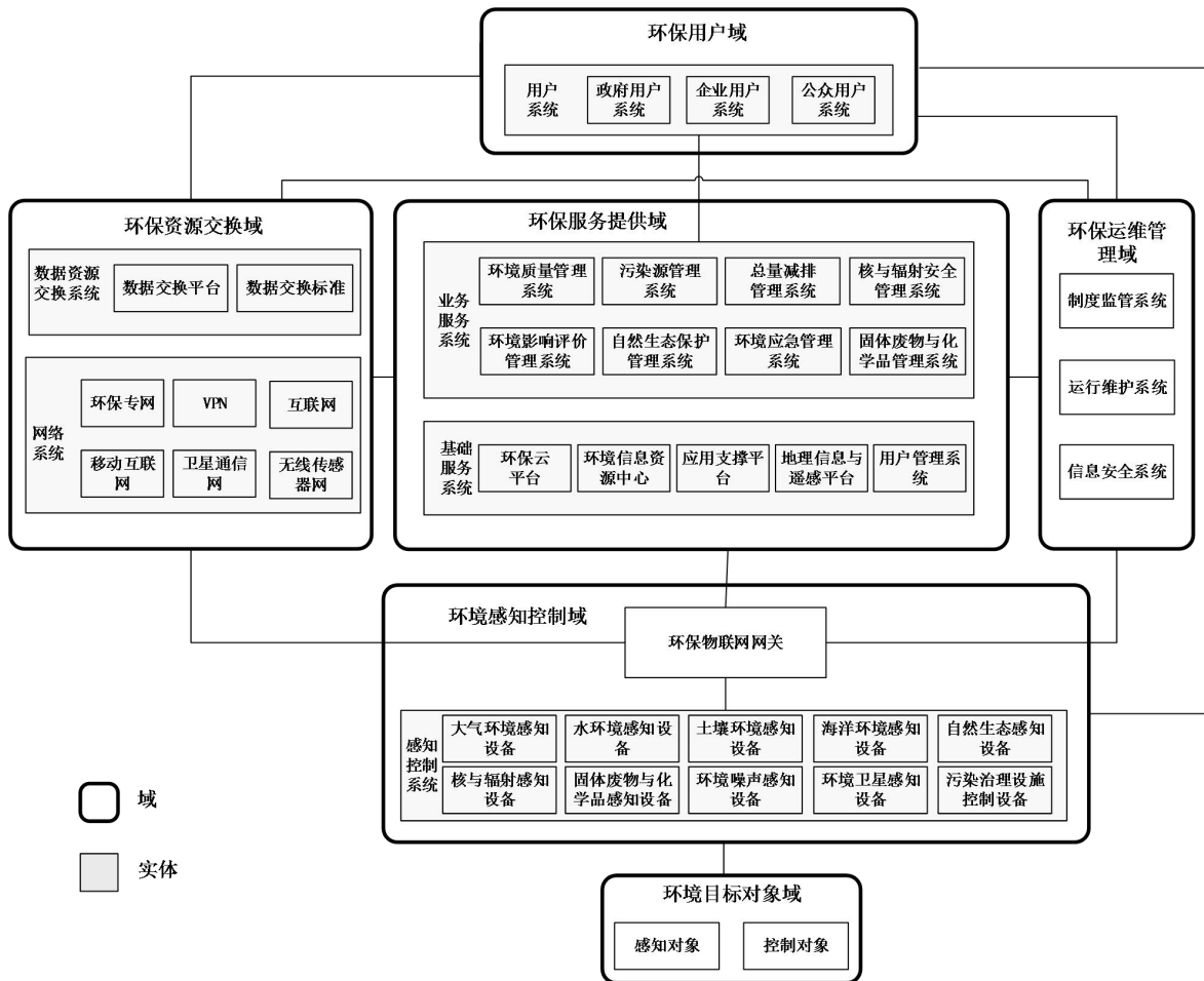
图2 环保物联网应用体系结构
