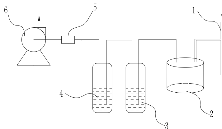
图 3-4 田间原位测定氨挥发的装置
